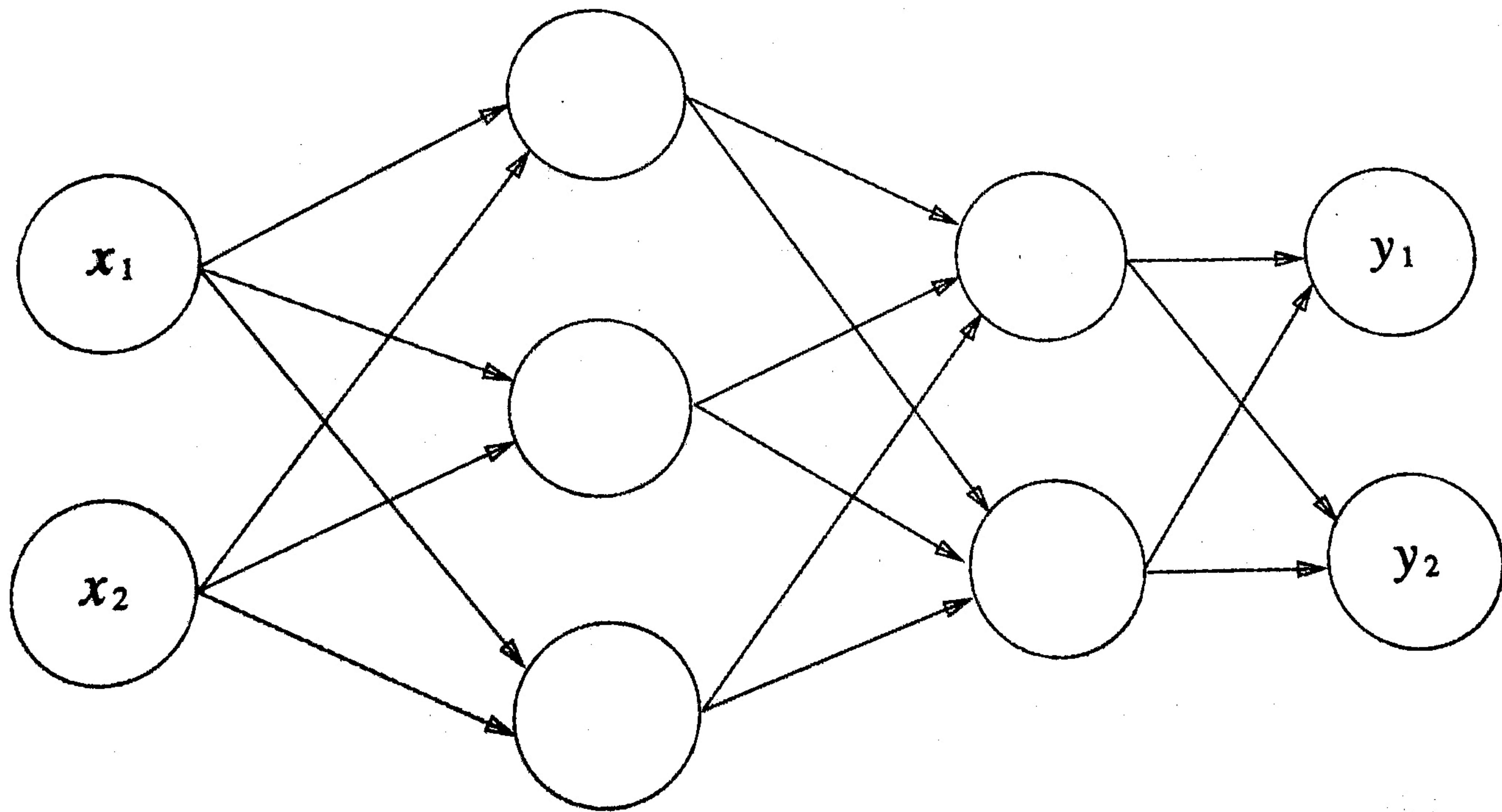
그림 3-15 3층 신경망 : 입력층(0층)은 2개, 첫 번째 은닉층(1층)은 3개, 두 번째 은닉층(2층)은 2개, 출력층(3층)은 2개의 뉴런으로 구성된다.
